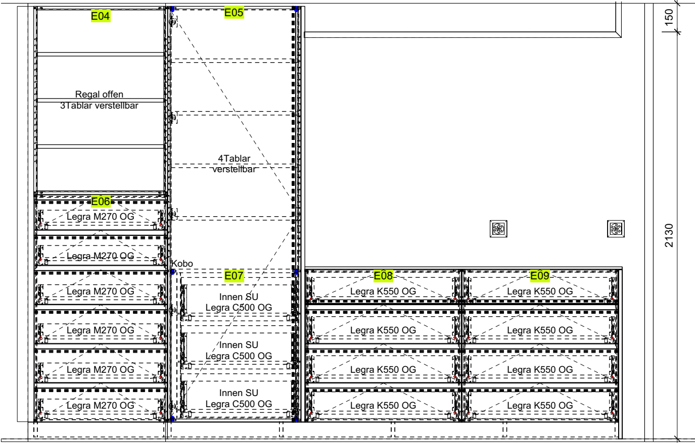
Ansicht 2
