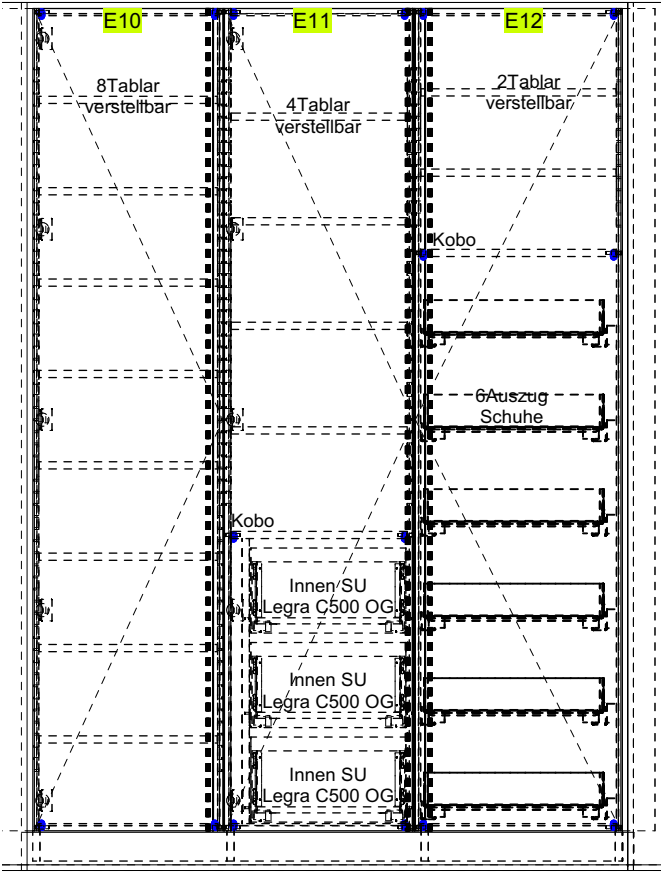
Ansicht 3
